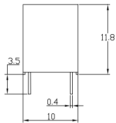
安装图
