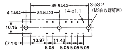
安装G7SA-4A2B时
