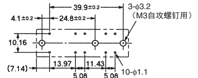
安装G7SA-2A2B时
